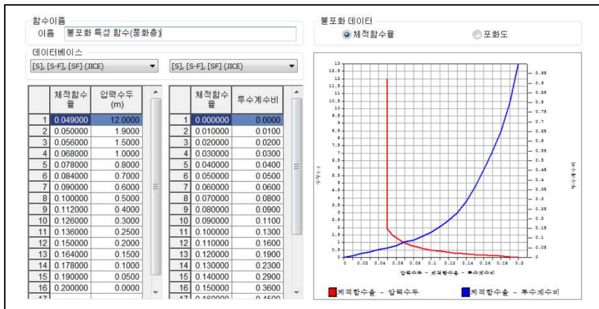
【그림 4.15】 압력수두-체적함수(포화도)-투수계수비 함수
