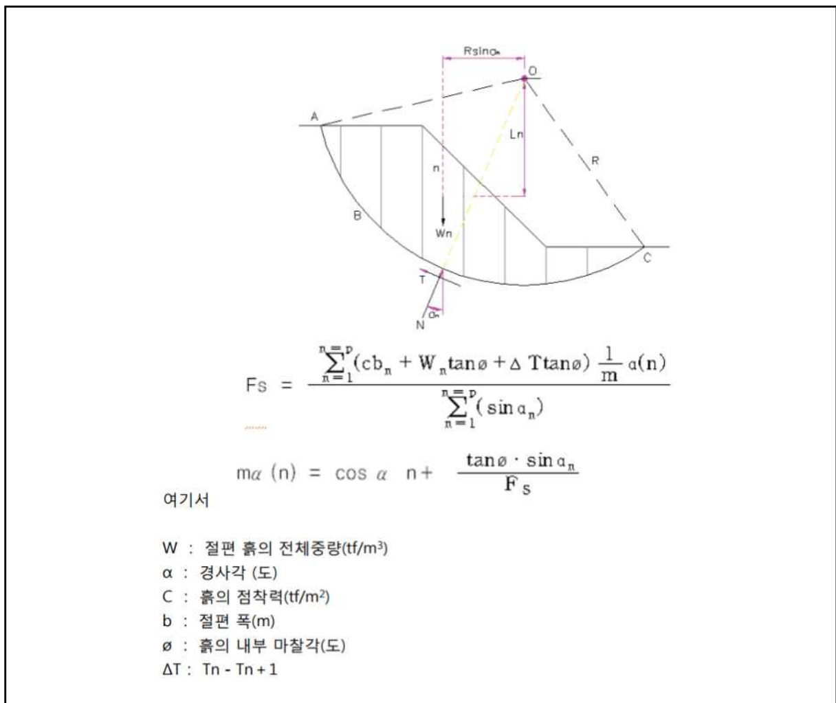
【그림 4.7】 Bishop의 안전율 계산식
