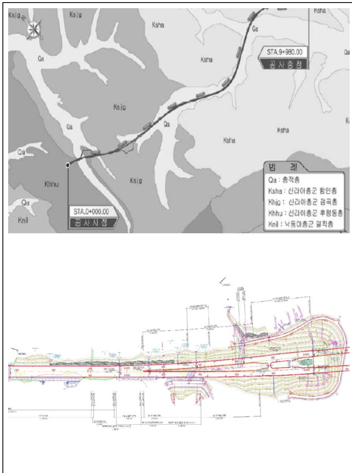
【그림 4.14】 영천절토04 검토대상 비탈면구간
