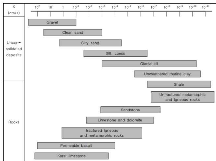
【그림 4.8】 퇴적물 및 암종별 투수계수(Freeze &amp; Cherry, 1979)
