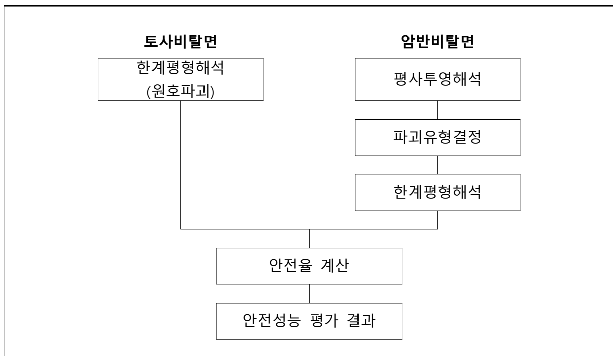
【그림 4.5】 구조안전성능 평가과정
