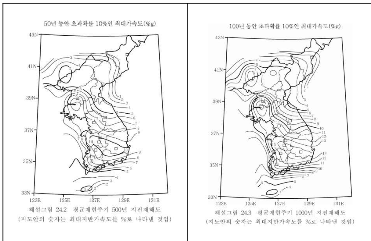
【그림 4.12】 평균재현주기 500년 및 1000년 지진재해도
